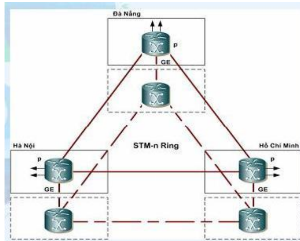
Hình 3. Sơ đồ khối mạng đường trục (Core)
