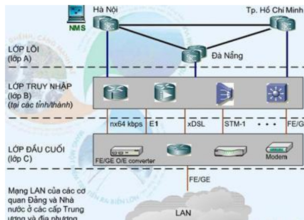
Hình 1. Sơ đồ cấu trúc phân lớp mạng TSLCD
